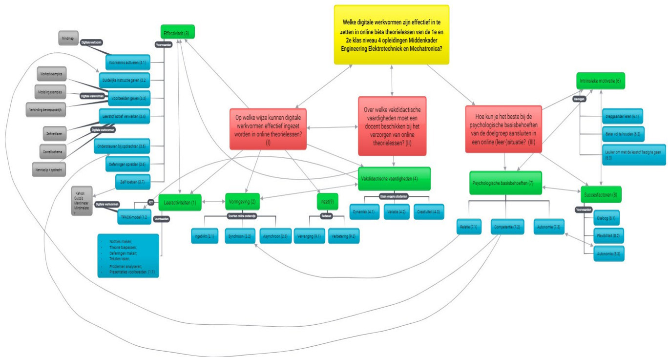
Figuur 1: Voorbeeld.concept.map
